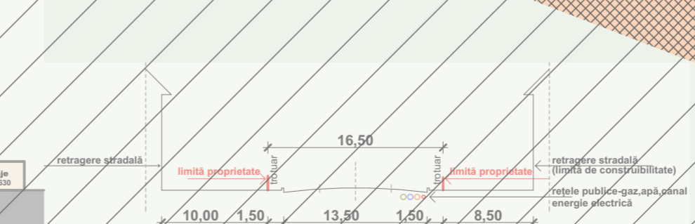
profil transversal strada Uzinei S1 sc 1:500
