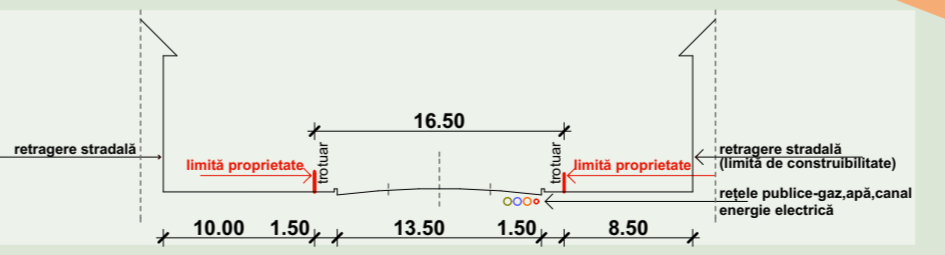
profil transversal strada Uzinei S1 sc 1:500
