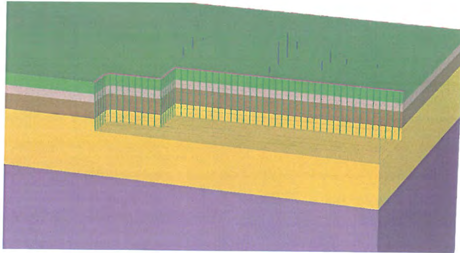
Excavație 7,00 m
