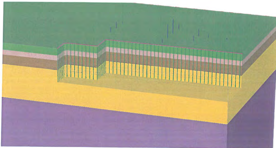
Excavație 8,00 m
