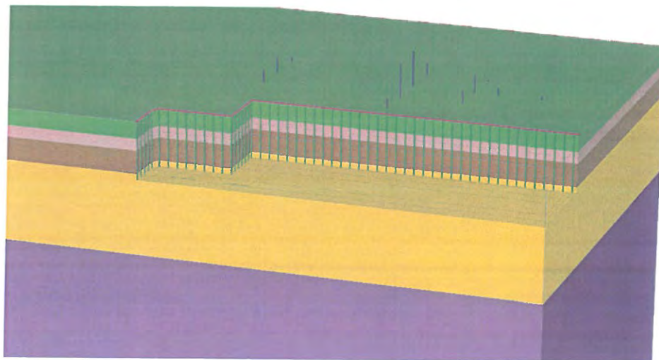
Excavație 5,00 m
