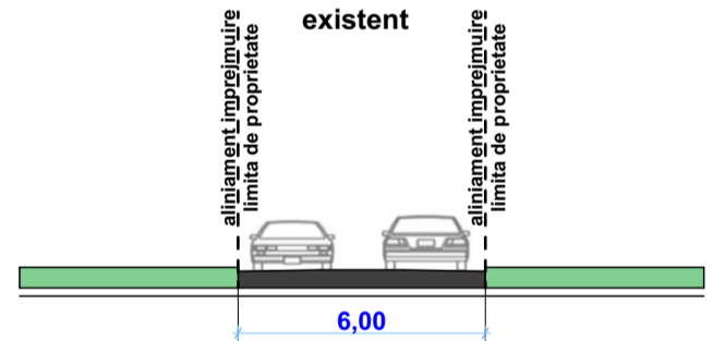
P2 - PROFIL STRADAL D.E.228 existent
