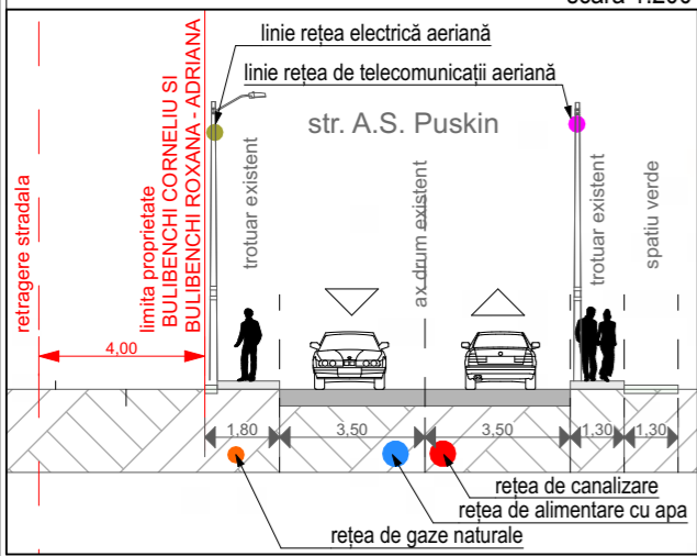
SECȚIUNE TRANSVERSALĂ 1-1, REȚELE EDILITARE, scara 1:200
