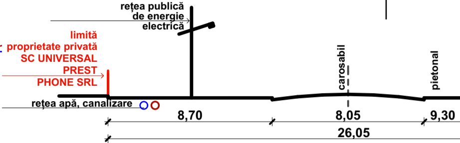
profil transversal existent str. Ion I.C. Brătianu sc. 1:200
