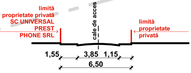
profil transversal existent cale de acces laterală sc. 1:200
