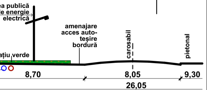
profil transversal propus str. Ion I.C. Brătianu sc. 1:200
