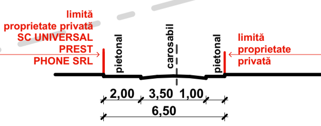
profil transversal propus cale de acces laterală sc. 1:200
