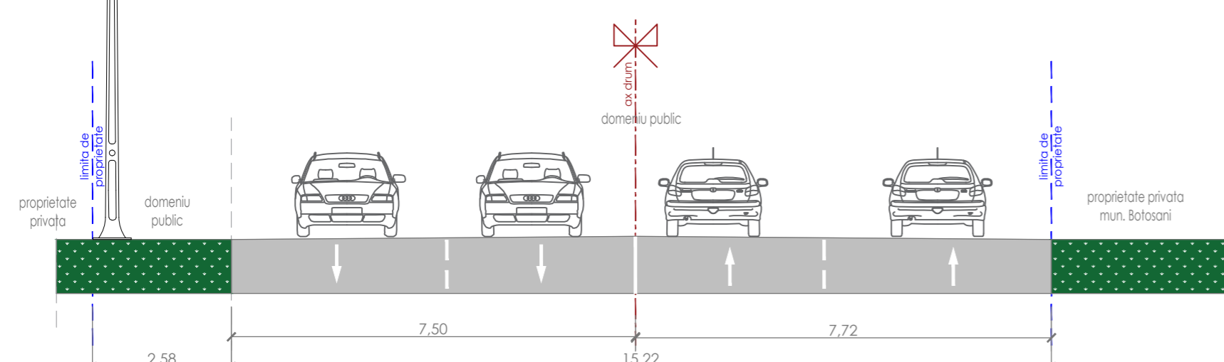
PROFIL STRADAL STRADA PACEA sc. 1 : 100
