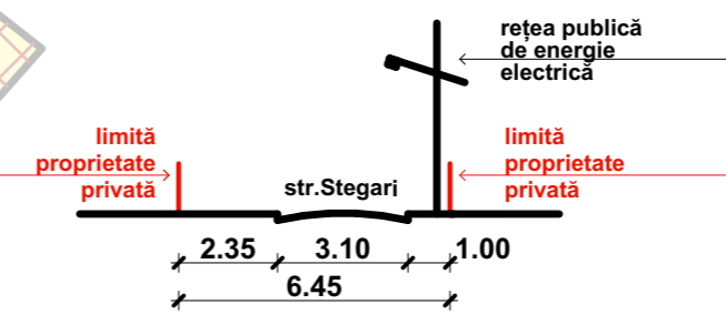
profil transversal existent str.Stegari NC/CF 69223 sc.1:200
