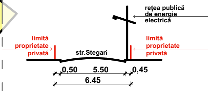
profil transversal menținut str. Stegari NC/CF 69223 sc.1:200
