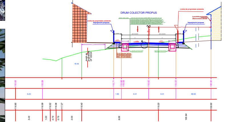
PI - PROFIL TRANSVERSAL Str. Pod de Piatra Drum modernizat
