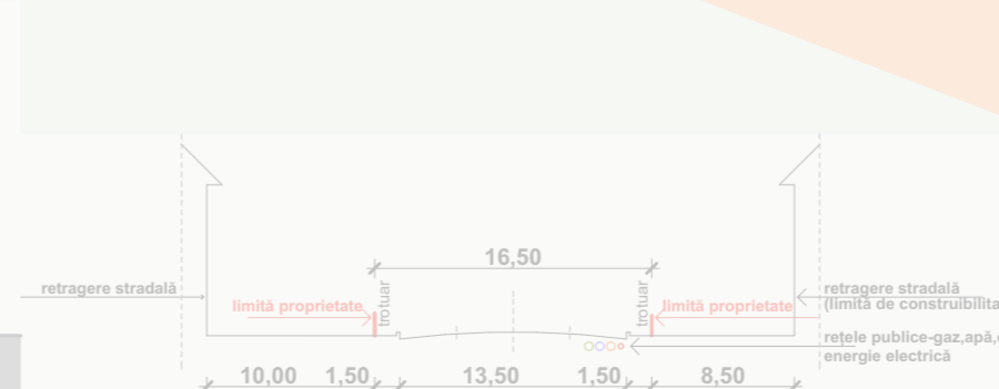
profil transversal strada Uzinei S1 sc 1:500
