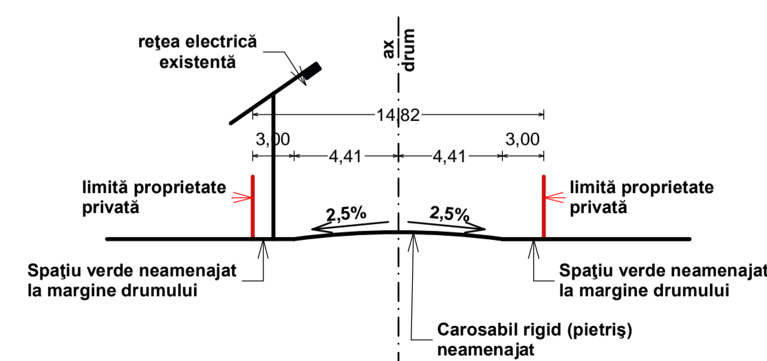
PROFIL TRANSVERSAL EXISTENT STRADA DRUMUL TĂTARILOR
